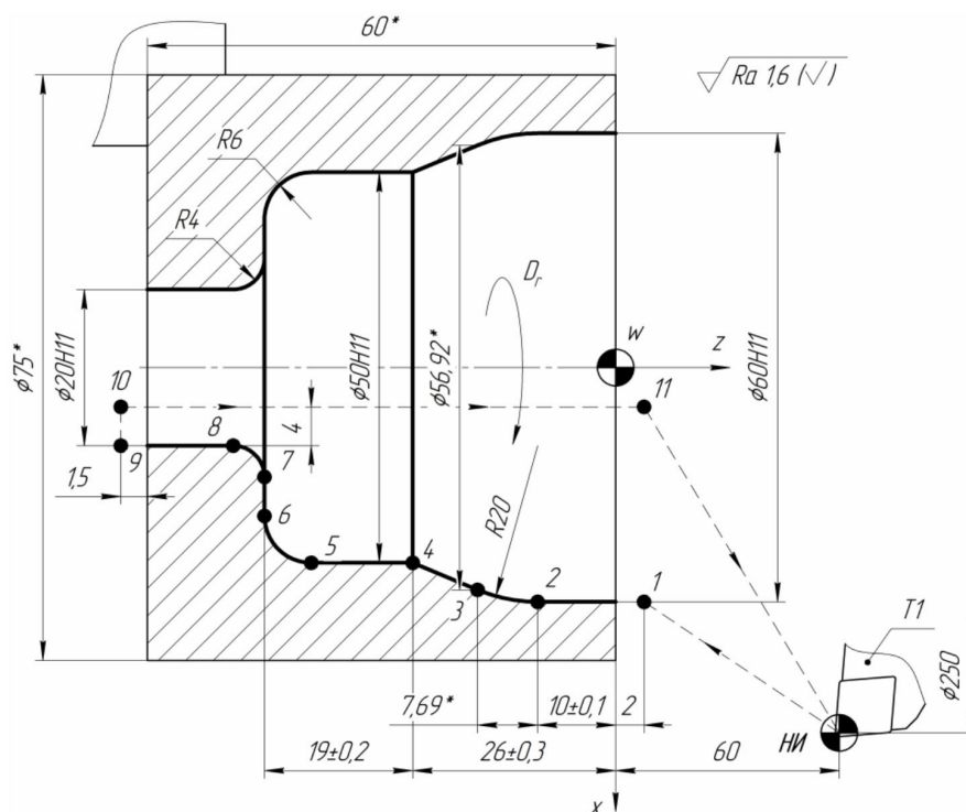
Рисунок 1. Эскиз расчетно-технологической карты
